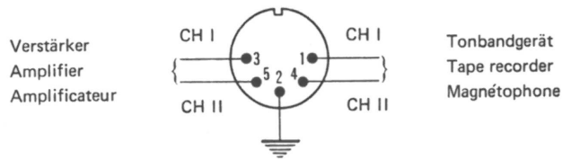
Sicht auf Stecker, Seite Lötflächen View on plug, solder lug side Vue de la fiche côté soudures
