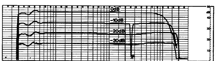
Fig. 8 Vier weergeefcurven met TDK SA C90, na bijstelling van de voormagnetisatie en met Dolby in. Let op de hogetonenafval bij 0 dB en de dip bij -10 dB
