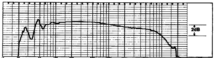
Fig. 6 Toepassing van Nakamichi EX C60-band, Dolby uit
