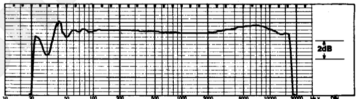
Fig. 5 Opn./weerg.curve na bijstelling van de voormagnetisatie op UDXL C90, Dolby uit, rechterkanaal
